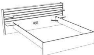
3580L280 : L235 x H98 x P217; Poids : 62 kg - Volume : 0,134m3; Nombre de colis : 3
