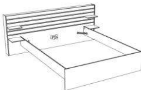
3580L260 : L223 x H98 x P217; Poids : 59 kg - Volume : 0,133m3; Nombre de colis : 3
