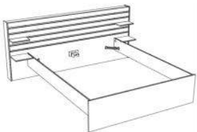
3580L240 : L203 x H98 x P217; Poids : 56 kg - Volume : 0,119m3; Nombre de colis : 2
